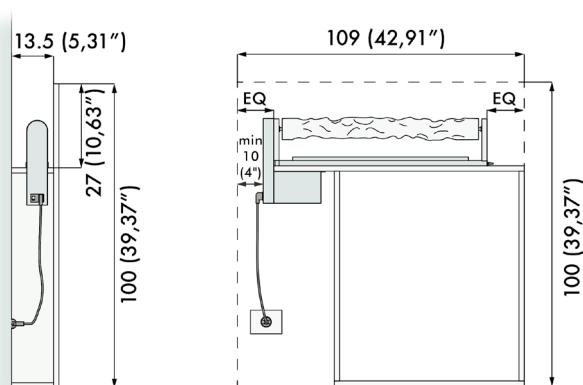
WW1: Main module 85 cm Modulo principale (33,46")
