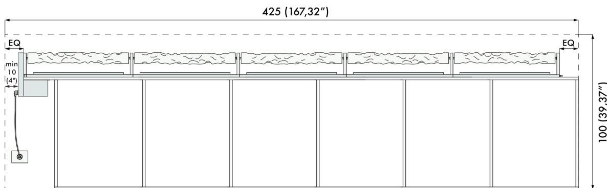
WW5: Main module + 4 additional modules 401 cm Modulo principale + 4 moduli aggiuntivi (157,87")
