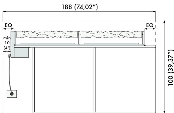
WW2: Main module + 1 additional module 164 cm Modulo principale + 1 modulo agg. (64,57")
