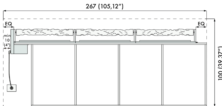
WW3: Main module + 2 additional modules 243 cm Modulo principale + 2 moduli aggiuntivi (95,67")
