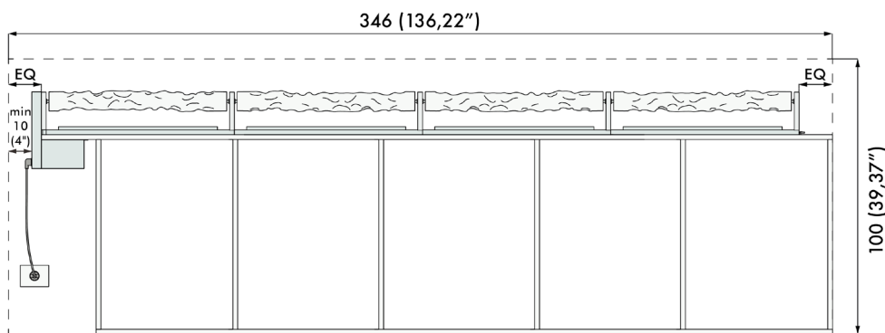
WW4: Main module + 3 additional modules 322 cm Modulo principale + 3 moduli aggiuntivi (126,77")
